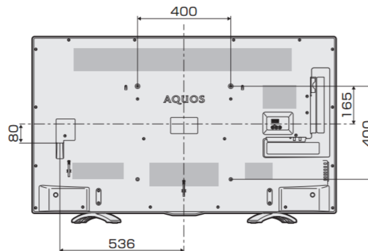
壁掛け金具取り付け部の寸法
