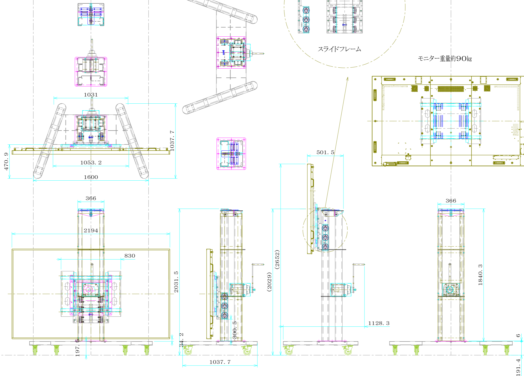
ウィンチ式1段昇降スタンド
